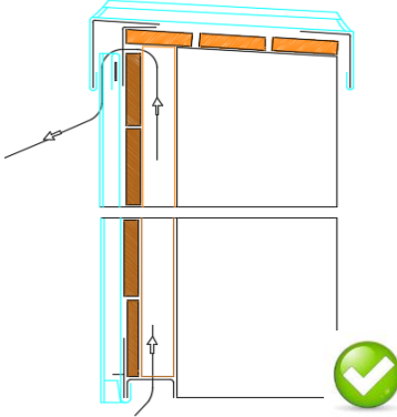
Standartlara uygun 2 cm havalandırma kesiti
