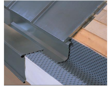
Havalandırmaz alt yapı üzerine delta VMZINC dere uygulama örneği
