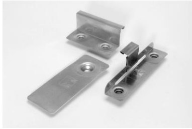
Sabit ve hareketli delta VMZINC paslanmaz çelik kenet klipsleri
