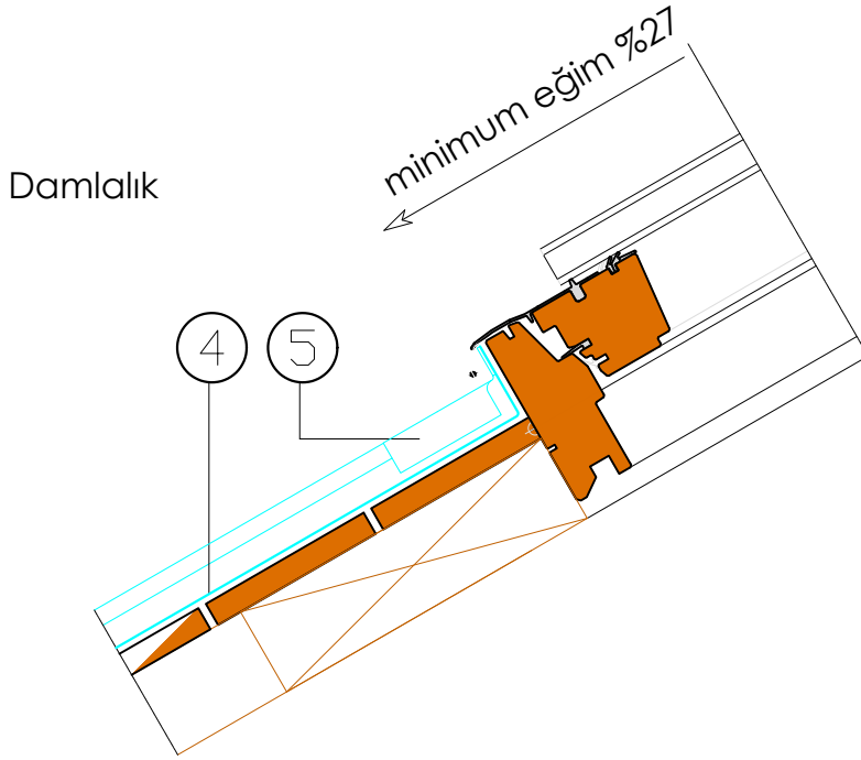
Boyuna kesit
