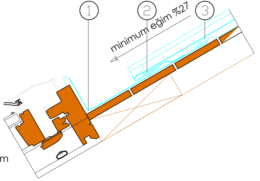
Boyuna kesit
